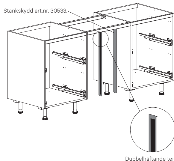
Dubbelhäftande tejp.
